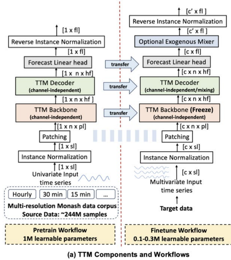
Σχήμα 3.3: Δομή του TTM από την δημοσίευση στο NeurIPS 2024 [1]
