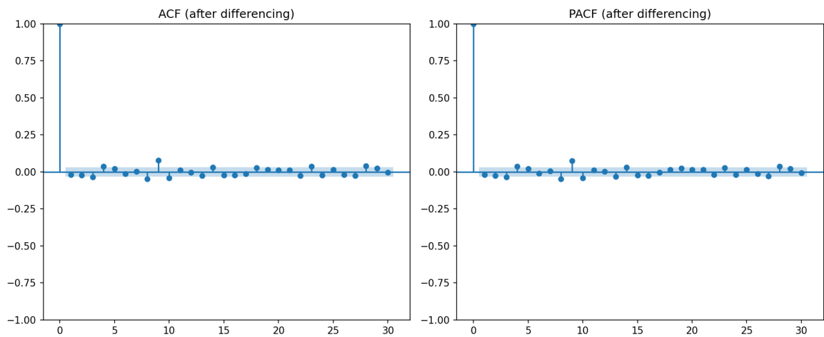
Σχήμα 6.2: Διαγράμματα ACF/PACF
