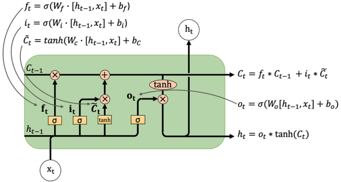
Σχήμα 3.1: Δομή LSTM
